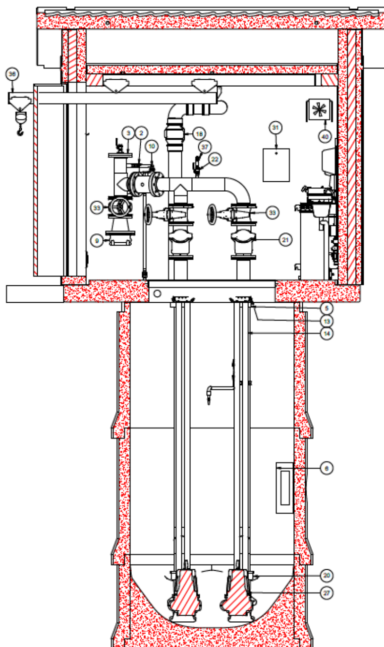
SEKTION D-D
